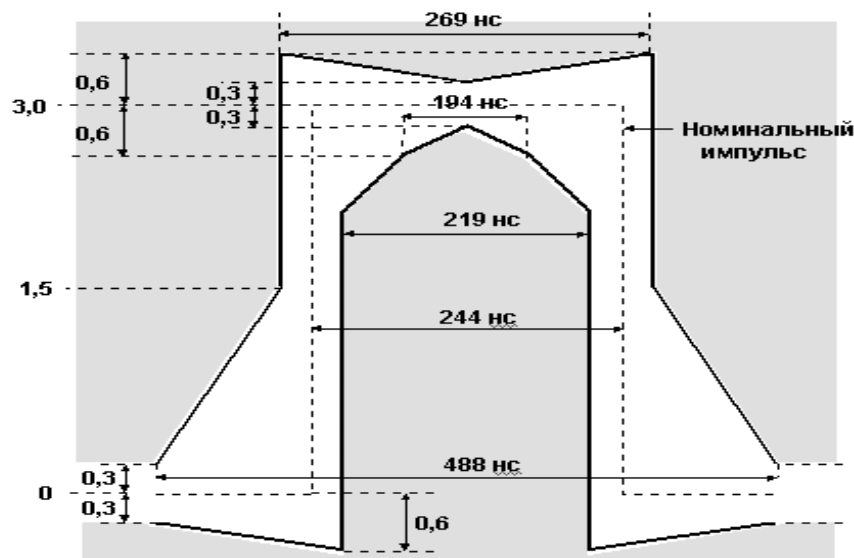
Рисунок 2. Форма и амплитуда импульсов синхросигнала 2048 кбит/с
