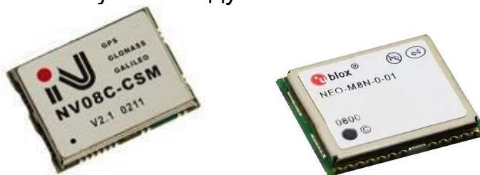
Рис. 2.1. Внешний вид модулей «NV08C-CSM и Ublox NEO»
